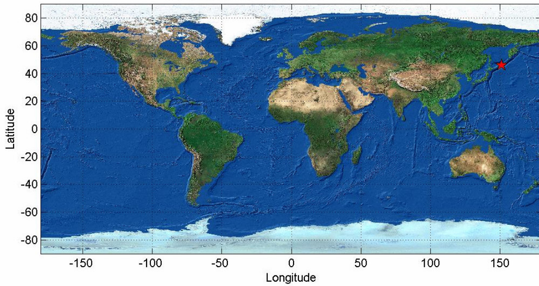
Epicenter Location (Kuril Islands 6.7 Moderate)
